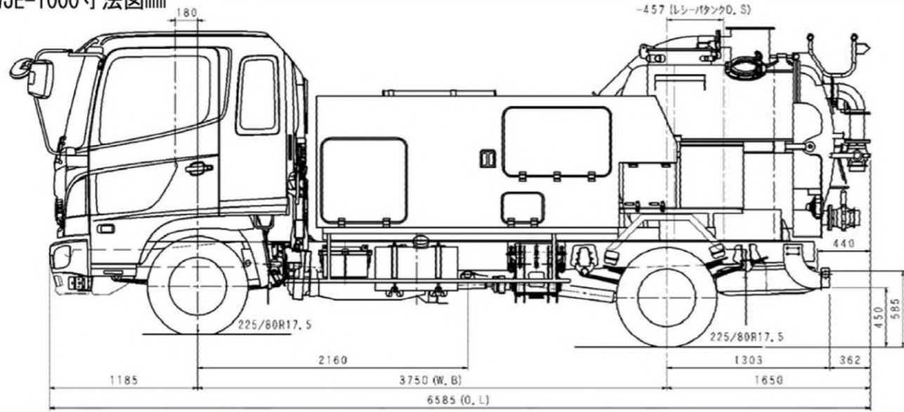
■WJE-1000寸法図mm
